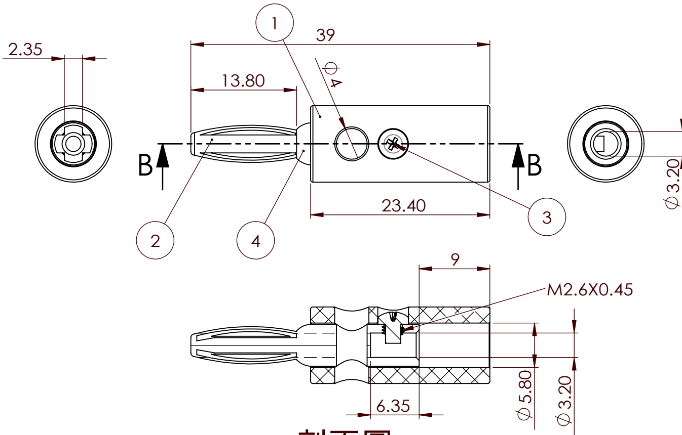
剖面圖 B-B
